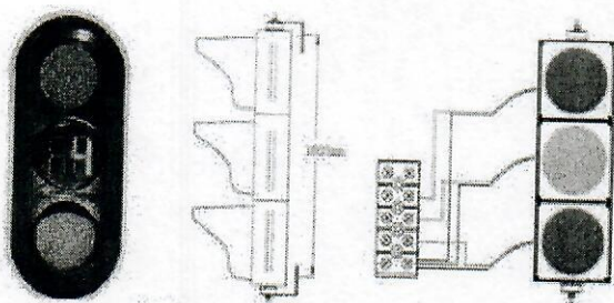
1.1. Lampă semafor pentru trafic auto
