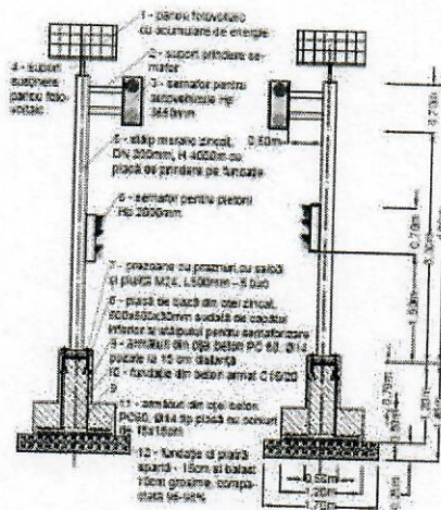
Fig. 11. Sistem de susținere instalat pentru semaforizare și fundare
